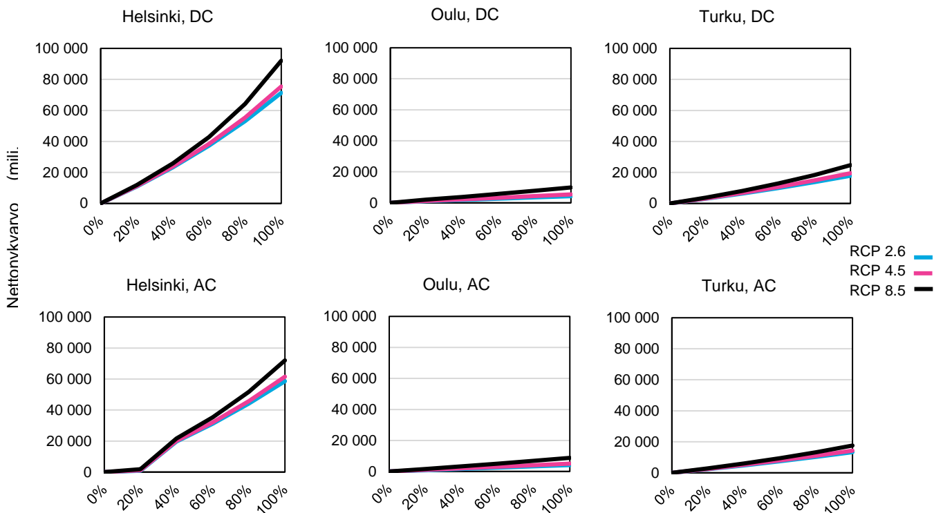
Kuva 4. Kaukokylmennyksen (DC) ja asennettavien ilmastolaitteiden (AC) nettonyökyarvo Helsingin, Oulun ja Turun kaupungeissa kylmennyksen piirissä olevan haavoittuvan populaation osuuden funktiona.
