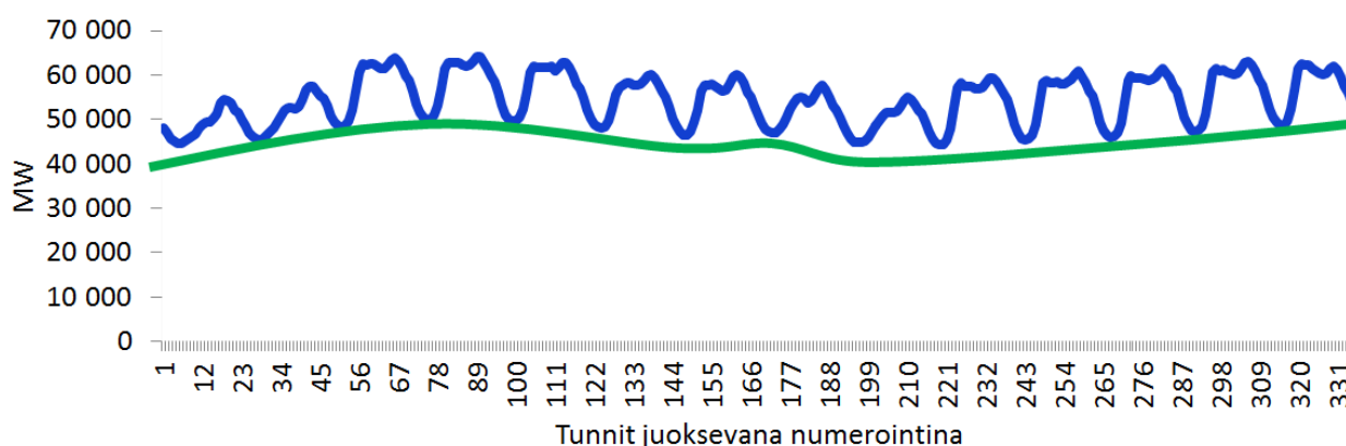
Kuva 7. Pohjoismaiden sähkönkulutus vuonna 1.1.2011-14.1.2011 (ylempi käyrä 22 ) ja esim. vesivoiman juoksutusta säatelemällä tasoitettu kulutus (alempi käyrä). Vesivoiman määrä on kuitenkin hyvin rajallinen, varsinkin huomioiden koko Euroopan tilanne.
